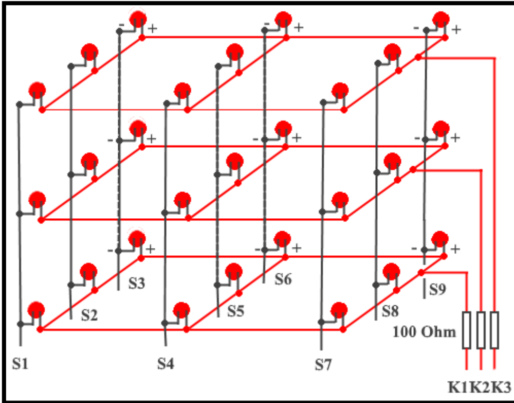
Resim 55. Led Küpü Şeması
