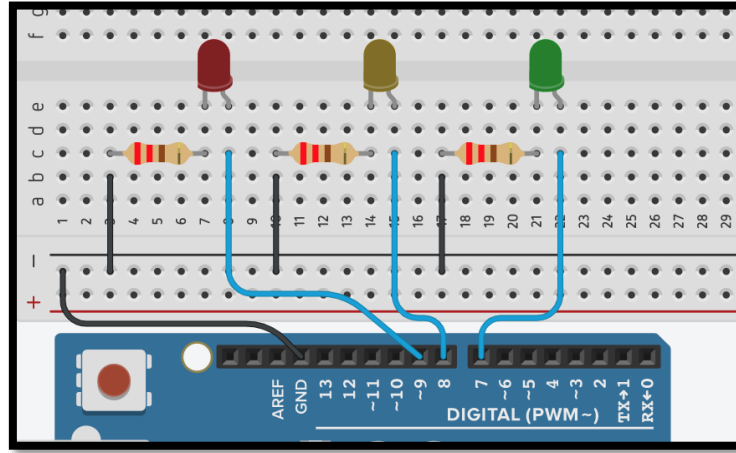
Resim 24. Örnek Devre Şeması
