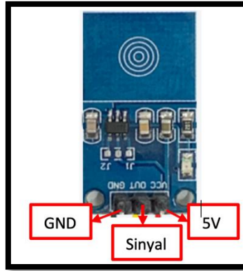
Resim 320. Dokunma Sensörü
