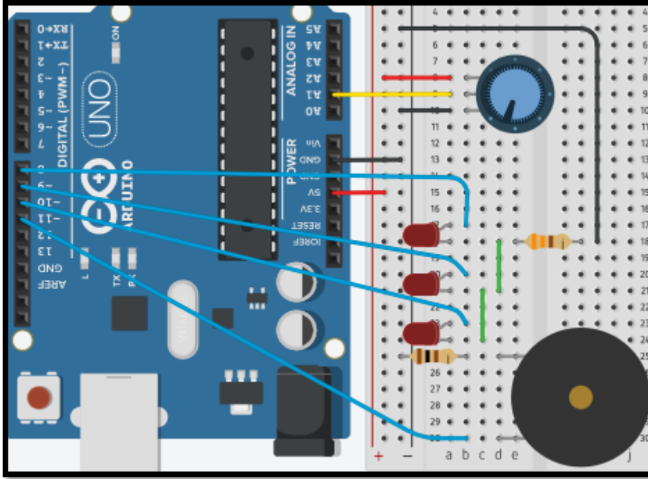
Resim 122. Örnek Devre Şeması
