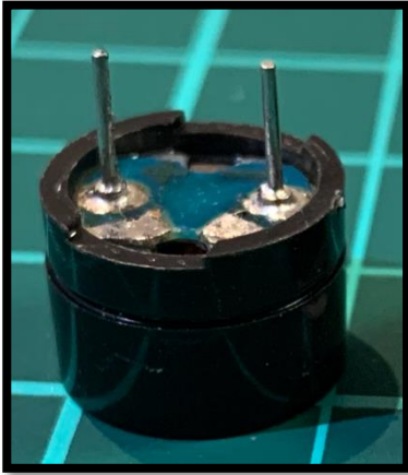
Resim 39. Pasif Buzzer
