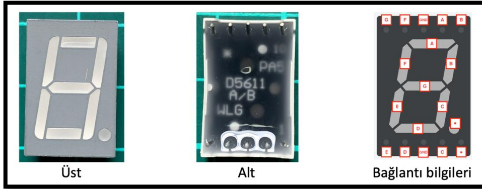
Resim 324. 7 Segmentli Gösterge
