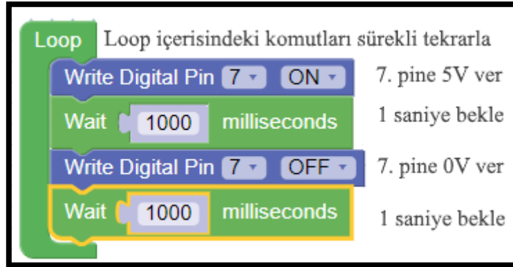
Resim 21. Örnek Program
