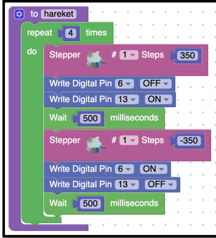
Resim 183. Hareket Fonksiyonu
