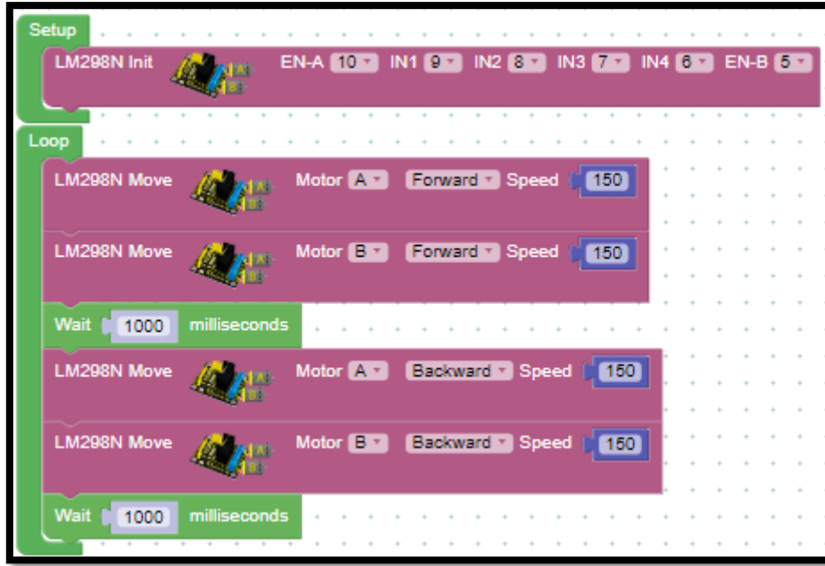
Resim 212. Örnek Program
