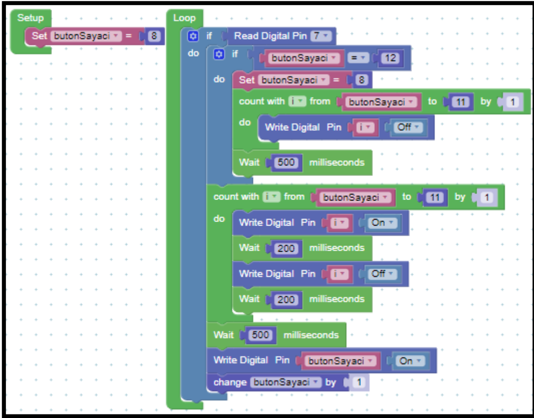
Resim 104. Örnek Program
