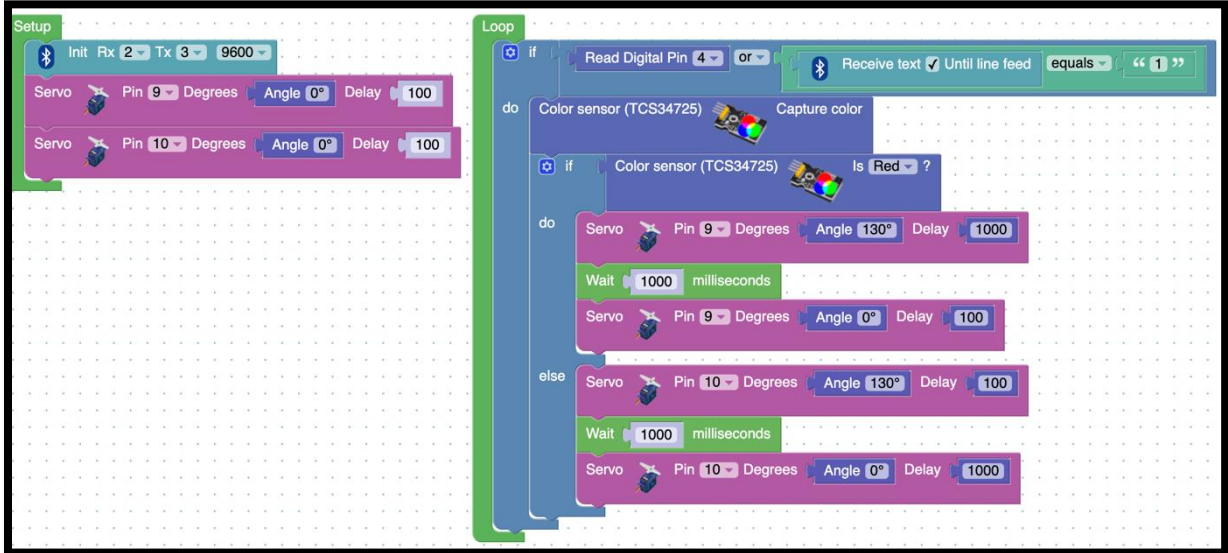
Resim 334. Örnek Program
