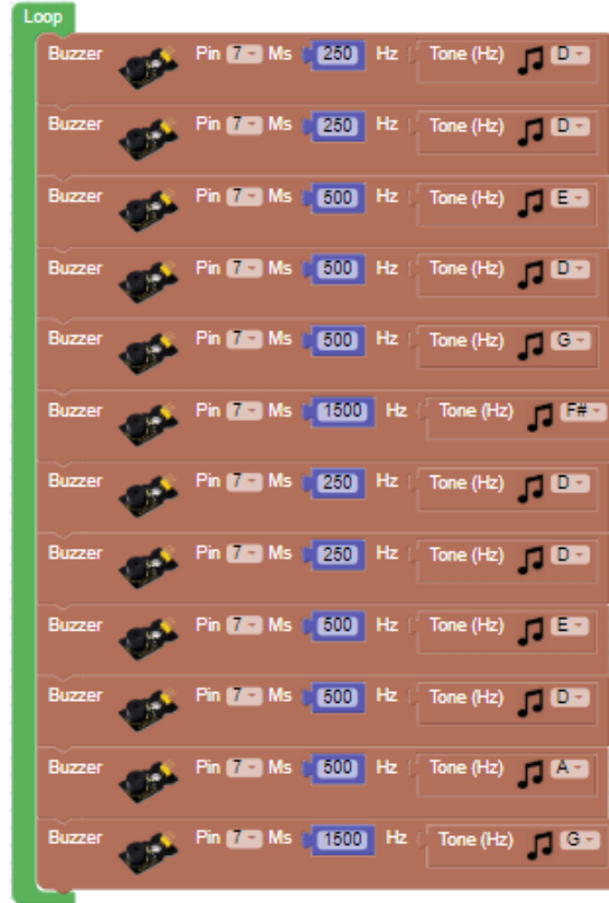
Resim 362. Örnek Program
