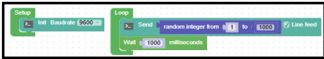
Resim 172. Örnek Program
