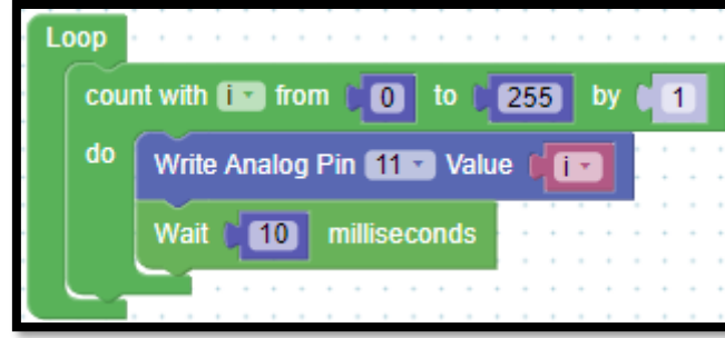
Resim 133. Örnek Program
