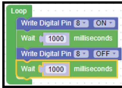
Resim 149. Örnek Program
