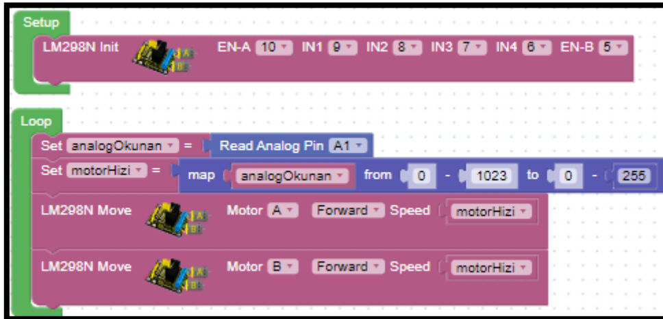
Resim 211. Örnek Program
