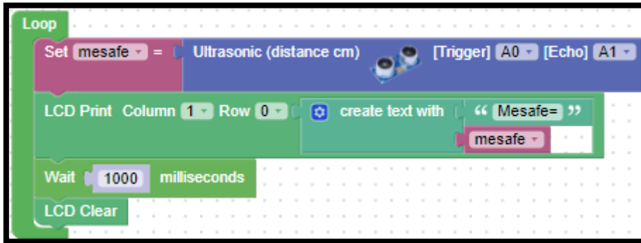
Resim 241. Örnek Program
