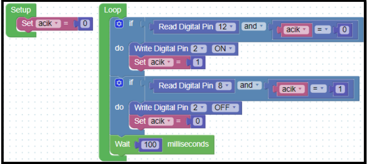
Resim 118. Örnek Program
