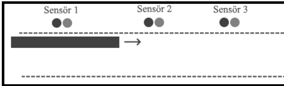
Resim 228. Yer Bildirimi
