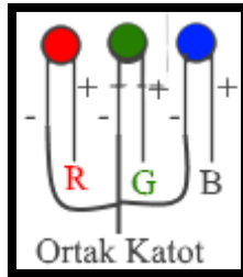
Resim 107. Katot RGB Led
