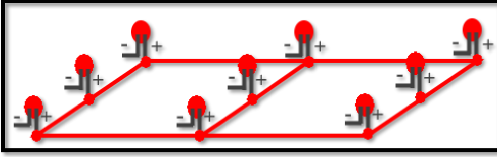
Resim 54. Led Küpü Üst Kat
