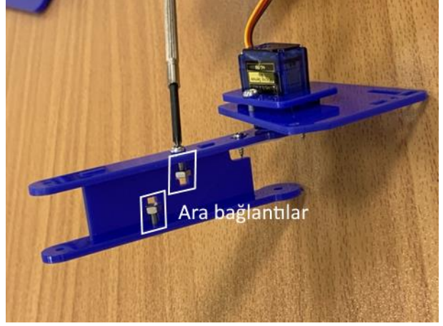
İki çubuğu birleştiren ara bağlantılar yapılır.
