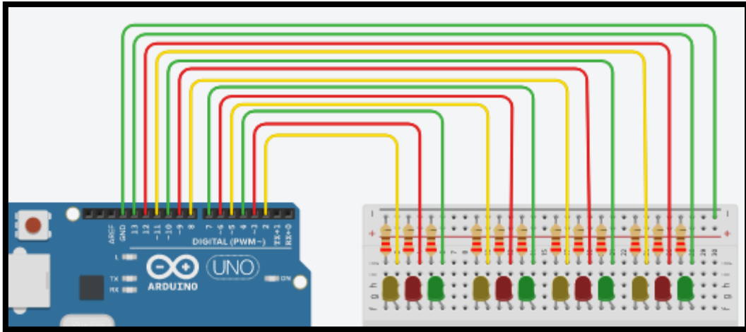
Resim 30. Örnek Devre Şeması
