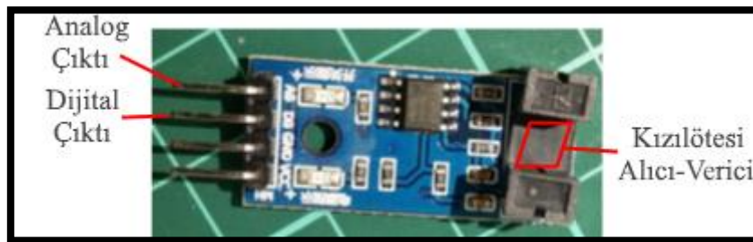
Resim 373. Kızılötesi Sensör
