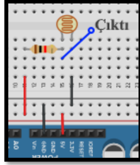
Resim 126. LDR Bağlantı 1
