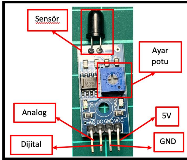
Resim 267. Alev Sensörü
