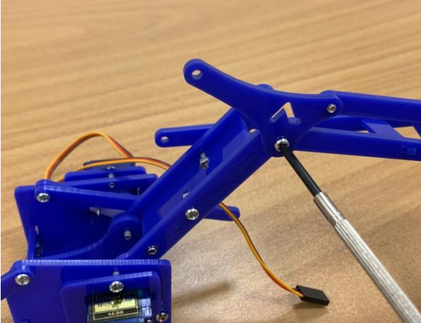
Birinci civata sıkılır.
