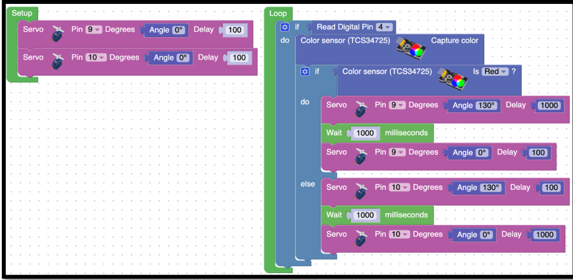
Resim 327. Örnek Program
