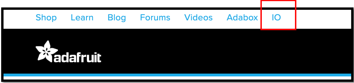
Resim 296 AdaFruit Girişi
