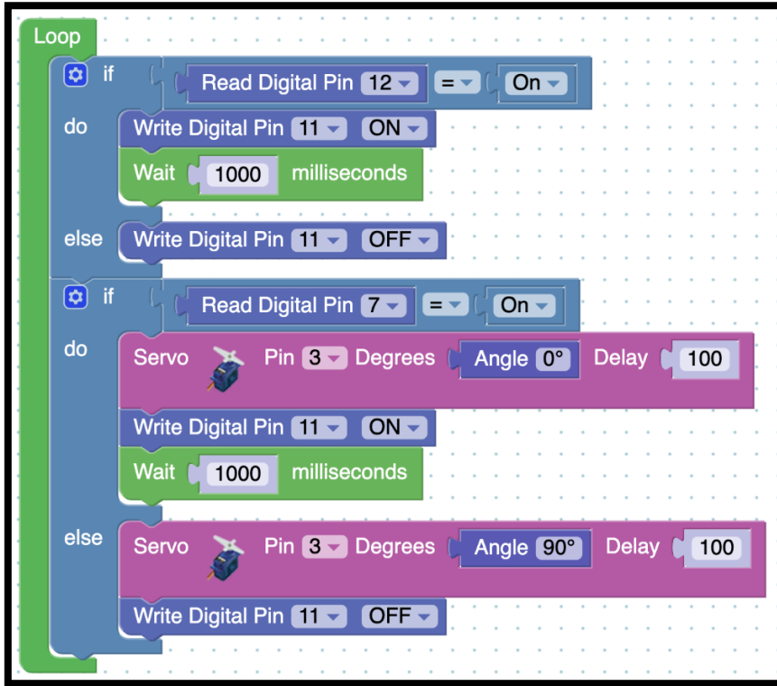
Resim 271. Örnek Program
