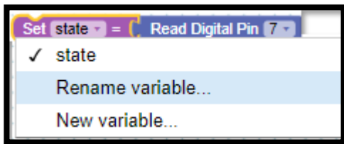
Resim 94. Değişken Oluşturma
