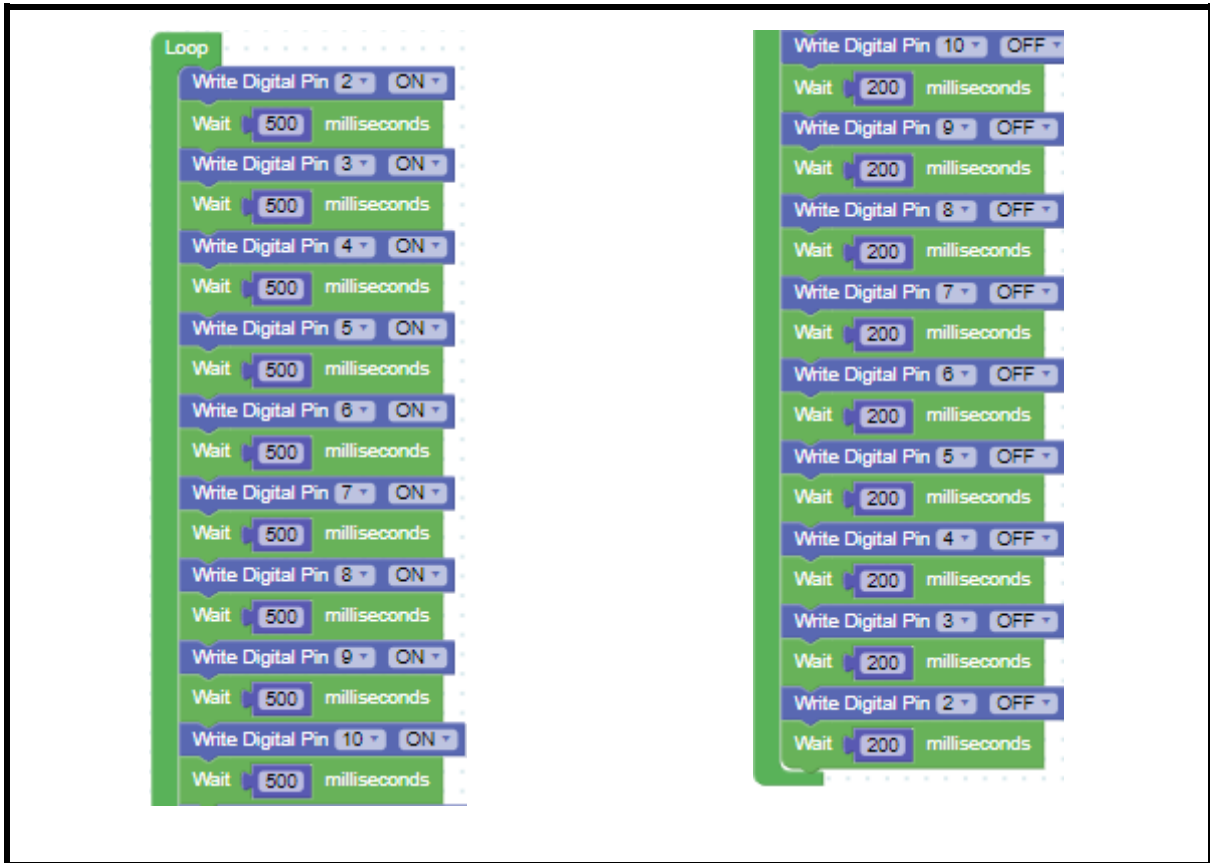
Resim 36. Örnek Program
