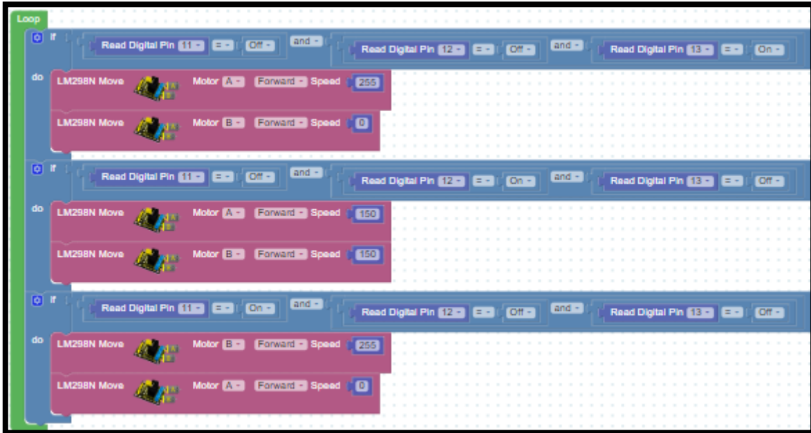
Resim 233. Örnek Program
