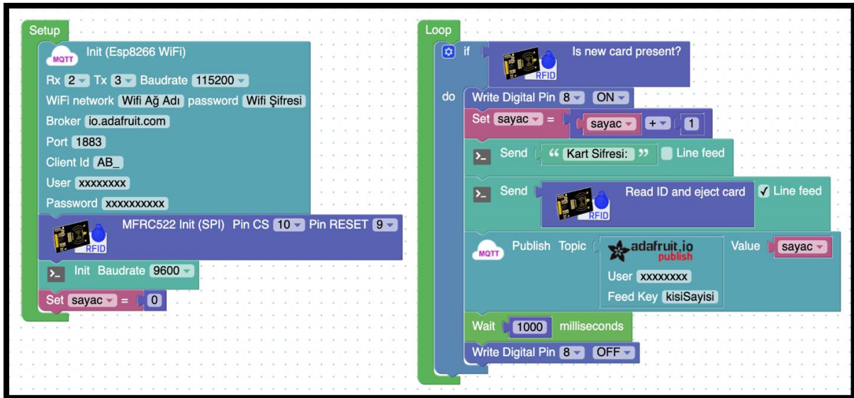
Resim 308. Örnek Program
