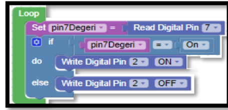
Resim 99. Değişkenli Kullanım
