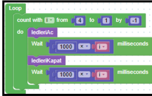
Resim 64. Örnek Program
