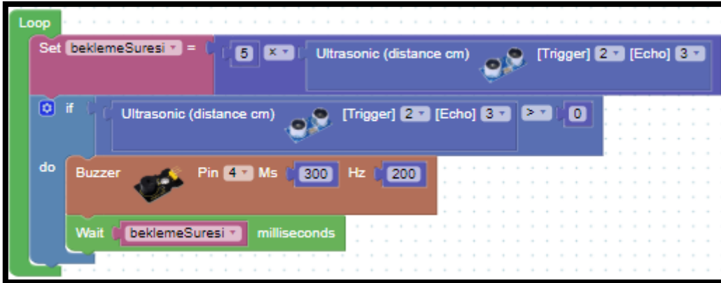
Resim 216. Örnek Program
