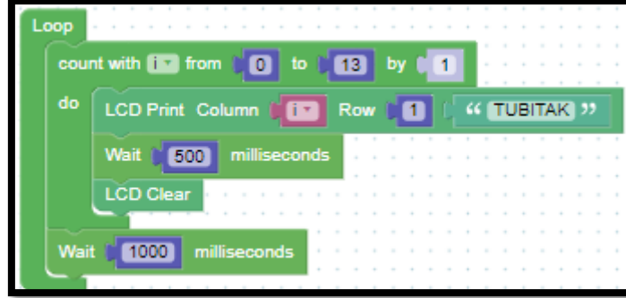
Resim 238. Örnek Program
