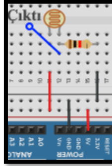
Resim 127. LDR Bağlantı 2
