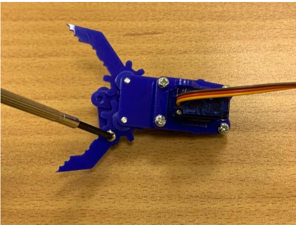
İki adet pulu baėlantı iin yerleřtirmeyi unutmayınız.
